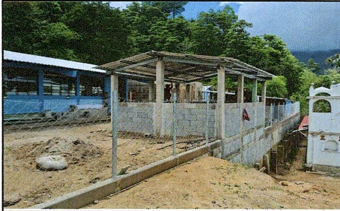
Foto 1: Terminación de muro de contención, cocina y circulación con postes de tubo y malla área frontal.
